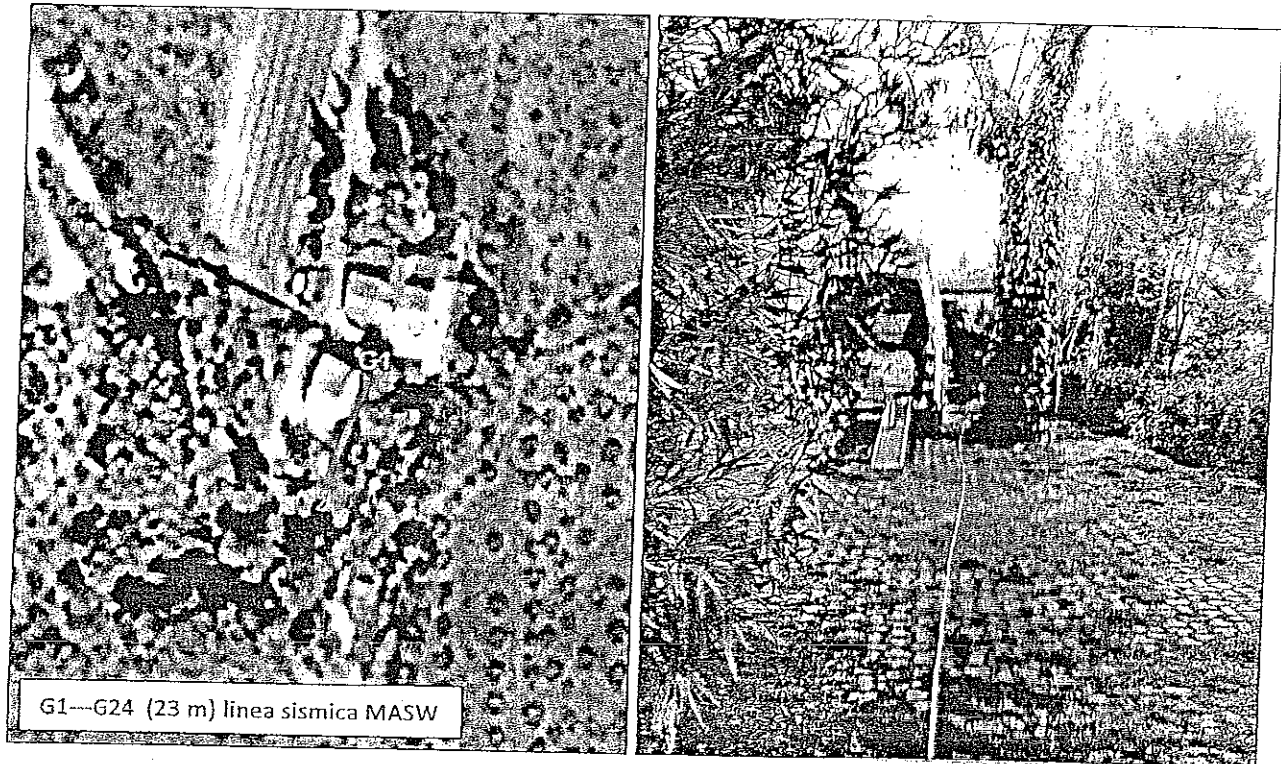
Fig.1: Ubicazione linea sismica masw
